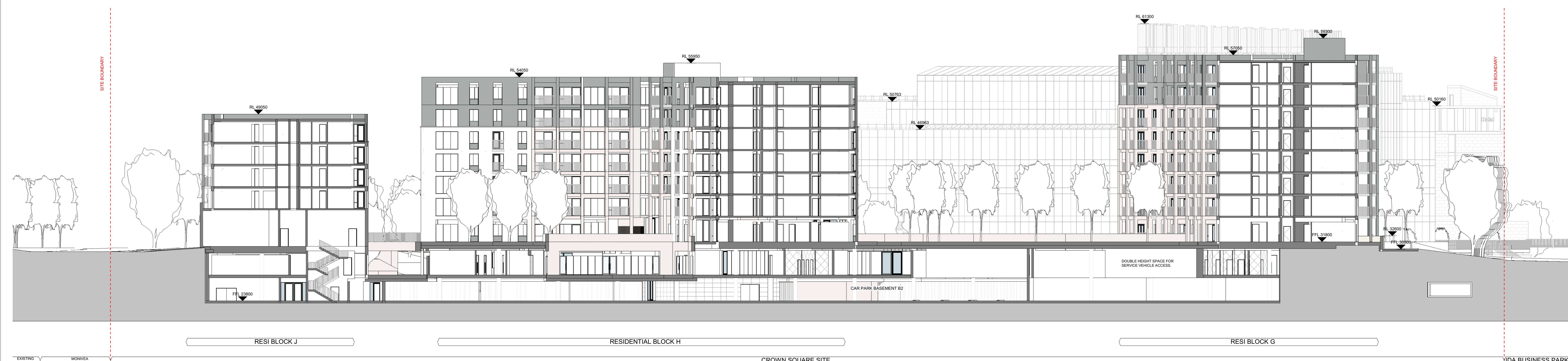
2 Site Section 7 1:200
