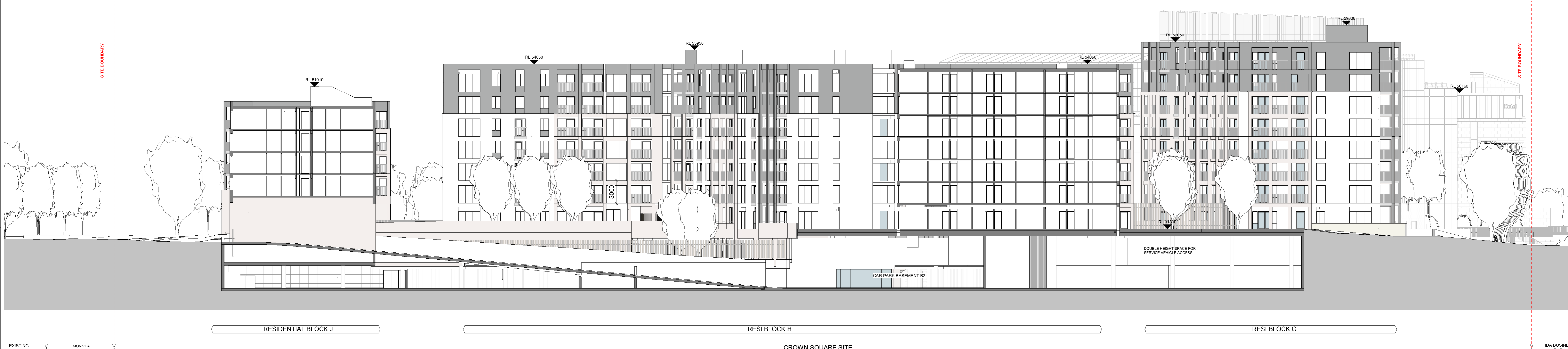
1 Site Section 6 1:200
